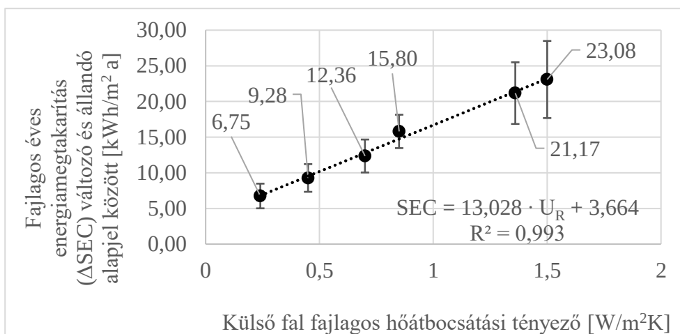
5.1. ábra Lakóépületek ( A=100-170 \text{ m}^2 , U_R= 0,32-0,987 \text{ W/m}^2K , A/V=0,59-1,1 \text{ m}^2/\text{m}^3 ) fajlagos éves megtakarítása
