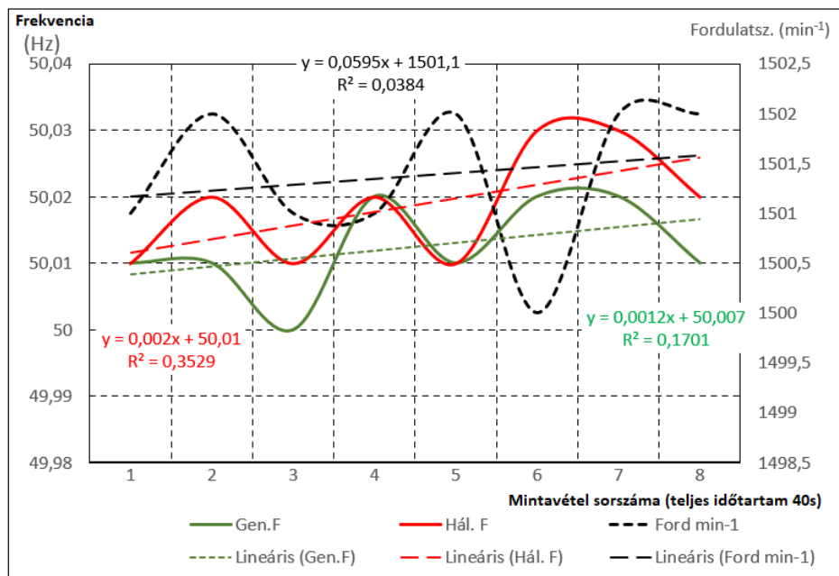
17. ábra Fordulat és frekvencia viszony - mintavétel 5 s-ként (saját ábra)
