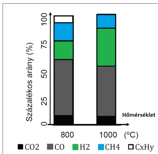
8. ábra Gázösszetétel változása 800/1000 °C-on, - G30 vegyes faapríték (MGI labor)
