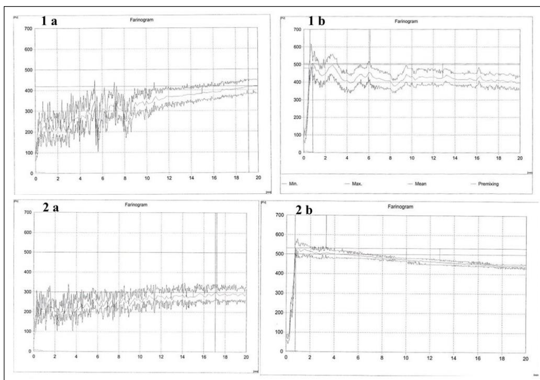
2. ábra: A predikciós modell segítségével kapott lisztkeverékek farinográfos görbéi (1.a: barnakenyér liszt hidrokolloid nélkül; 1.b: barnakenyér liszt hidrokolloiddal; 2.a: fehérkenyér liszt hidrokolloid nélkül; 2.b: fehérkenyér liszt hidrokolloiddal)
