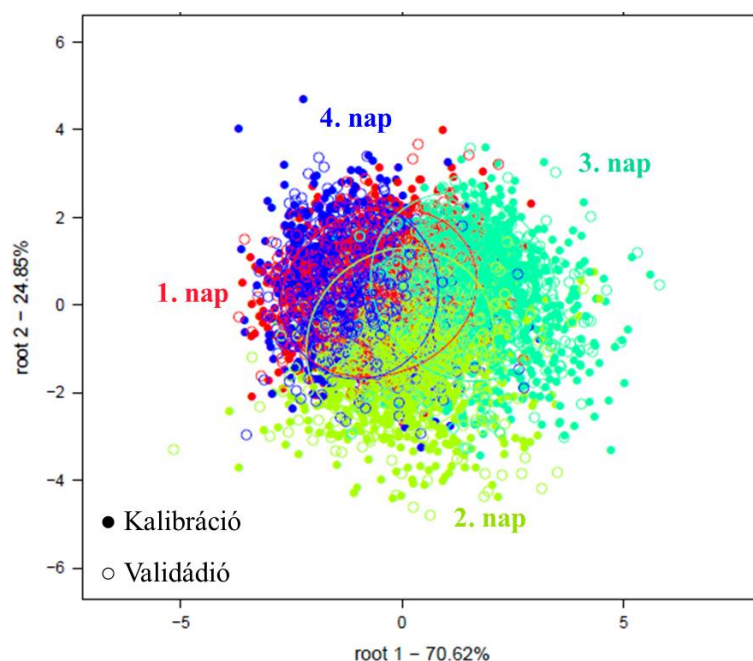
7. ábra: A vizsgált kenyérmintk tárolási időtartam szerinti LDA eredmények kiugró érték kezelés, simítás és sgol-2-13-1 előkezelés után (n=8390, NrPC = 30)
