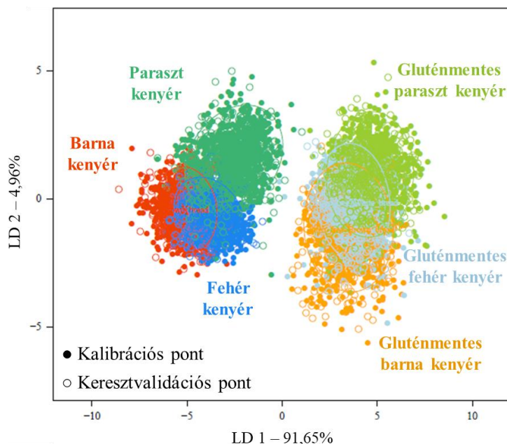
5. ábra: Kenyértípus szerinti LDA eredmények kiugró érték kezelés, simítás és sgol-2-13-1 előkezelés után (N = 8390, NrPC = 30)
