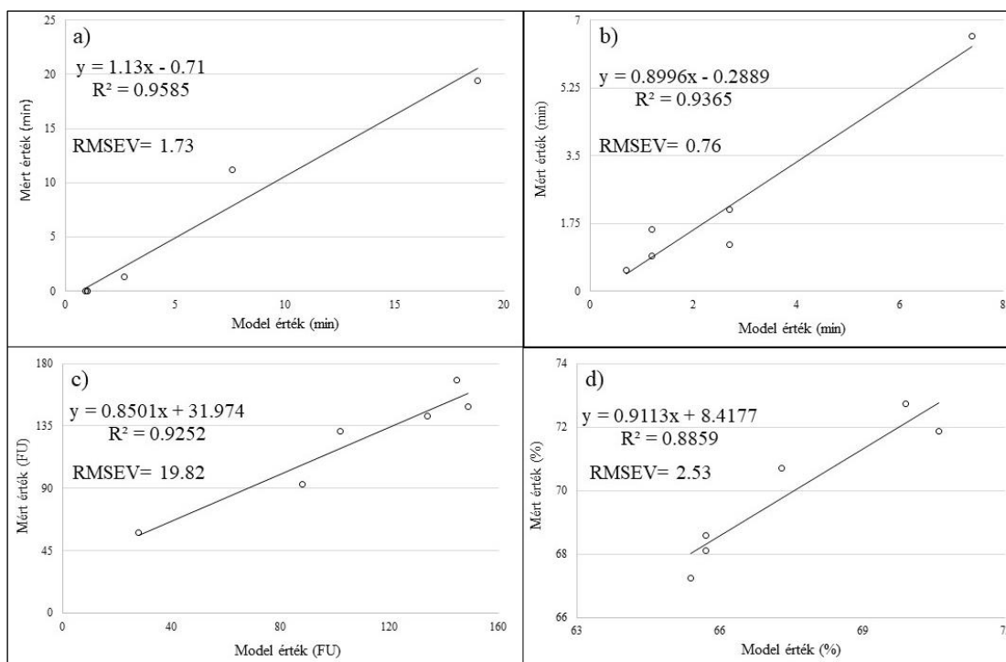
46. ábra: Validációs mérés eredményei (a: tészta kialakulási idő; b: stabilitás; c: ellágyulás; d: vízfelvétel)
