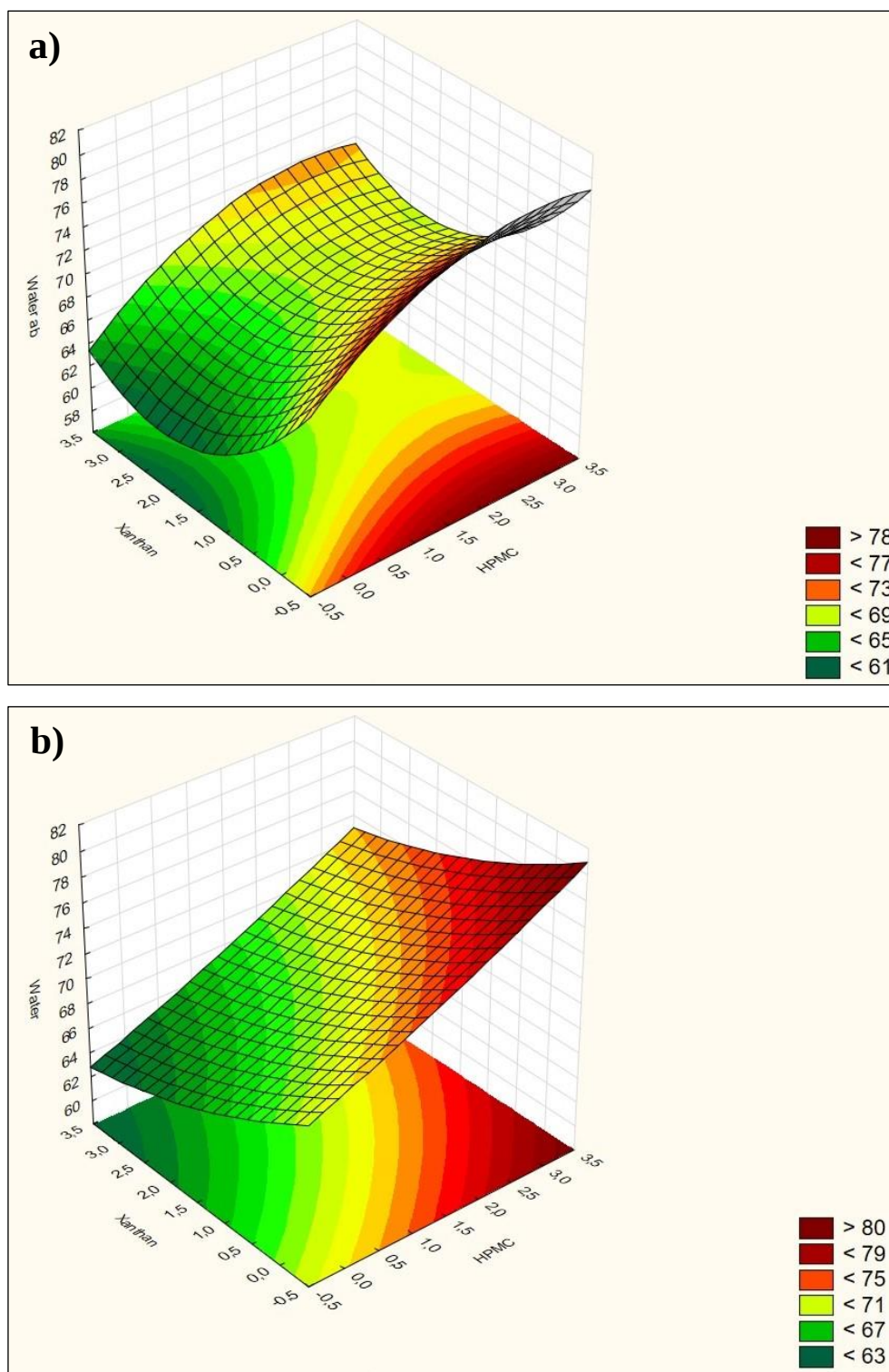
44. ábra: Az alapanyagok kombinációinak hatása a vízfelvételre (a: barnakenyér liszt; b: fehérkenyér liszt)
