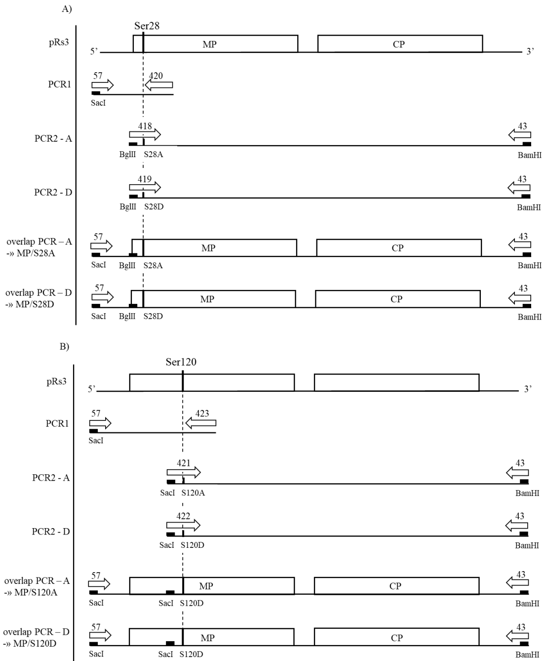
4. ábra. Az A) MP/S28A, MP/S28D, és B) MP/S120A, MP/S120D fertőzőképes klónok előállításának sematikus ábrája. A nyilak a primereket, míg a fekete téglalapok a bevitt restriktációs hasítóhelyeket jelölik.
