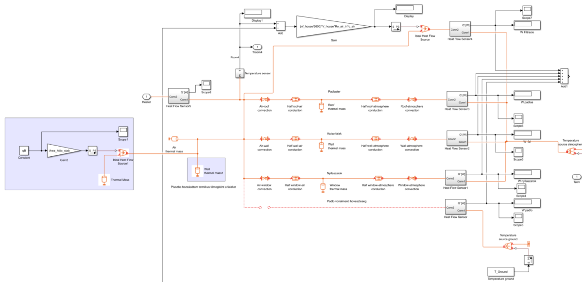
3.20. ábra A vizsgált épület lakóterének energetikai modellje MATLAB/Simulink környezetben A jobb áttekinthetőség miatt nagyobb részletben a 3.21. ábra a vonalmenti hőátbocsátás, a 3.22. ábra a filtráció modellezését mutatja be.
