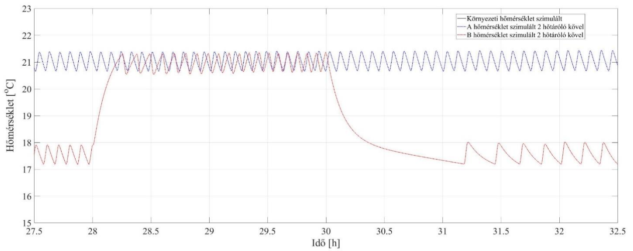
M3.21. ábra A és B kisminta modell hőtároló tömeg szimuláció 2. részlet
