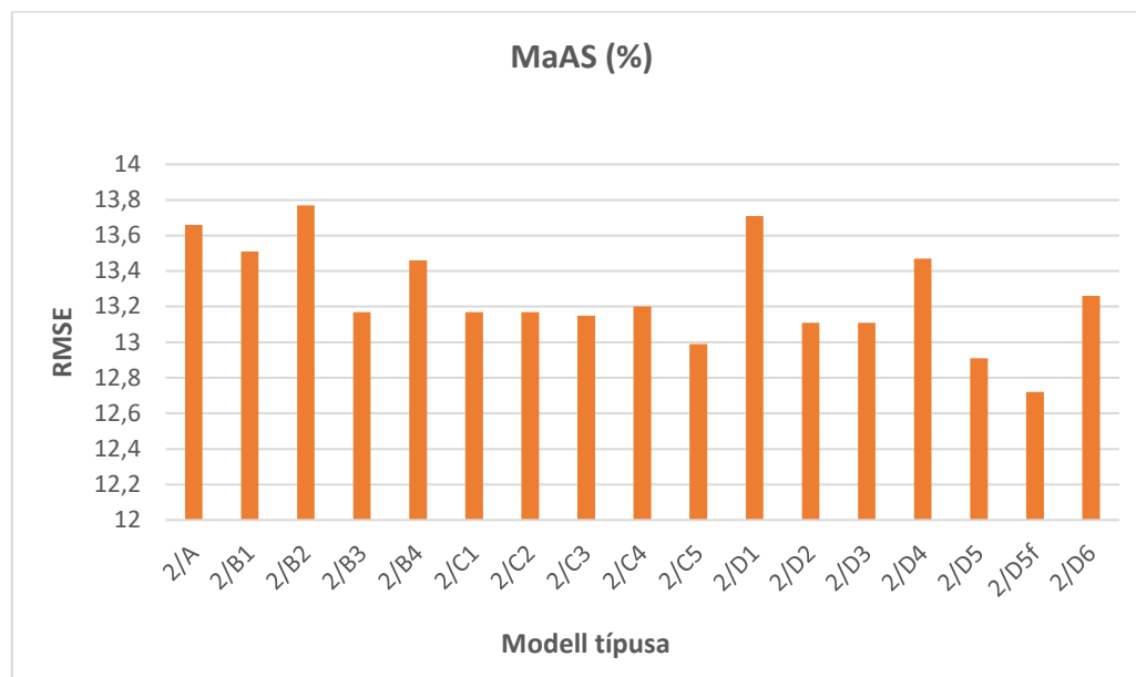
27. ábra: A makroaggregátum-stabilitást becsülő 2-es típusú, humuszminőség változókat is tartalmazó modellek hibája (RMSE)
