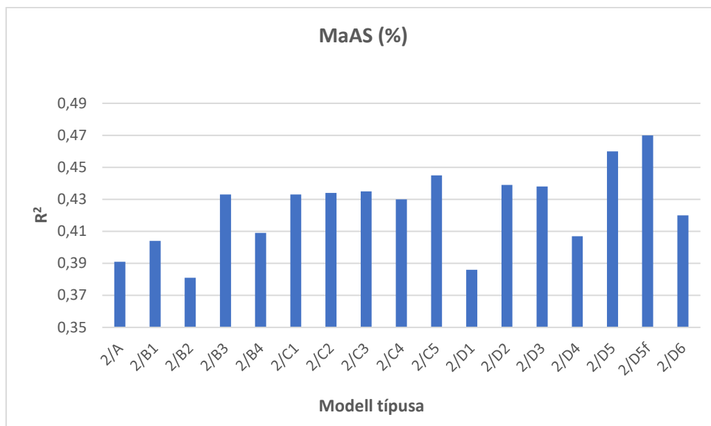
26. ábra: A makroaggregátum-stabilitást becsülő 2-es típusú, humuszminőség változókat is tartalmazó modellek statisztikai becselő pontossága ( R^2 )
