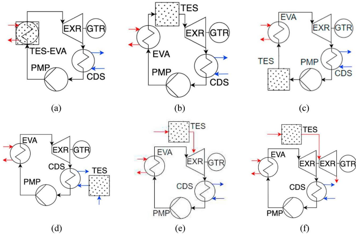
Fig. 2.14. TES-ORC configuration (Daniarta et al., 2023)
